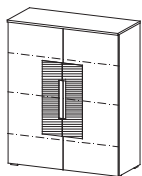
CU-K2 komoda W: 1235, S: 1000, G: 432
