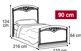
Bed "Curvo Fregio" 90x200 cm Letto "Curvo Fregio" 90x200 cm Vol. 0,25 kg 37,20 Box 3
