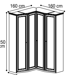
Composition X 62 Composizione X 62 Vol. 0,98 kg 216,40 Box 17
