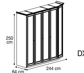
Composition X 10 Composizione X 10 Vol. 1,09 kg 232,70 Box 18
