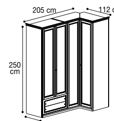
Composition X 44 Composizione X 44 Vol. 0,87 kg 235,20 Box 16
