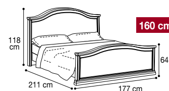
Bed "Gendarme" 160x200 cm Letto "Gendarme" 160x200 cm Vol. 0,42 kg 50,80 Box 3
