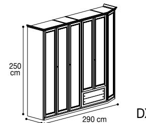
Composition X 04 Composizione X 04 Vol. 1,19 kg 283,90 Box 21
