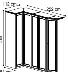
Composition X 65 Composizione X 65 Vol. 1,05 kg 250,50 Box 17
