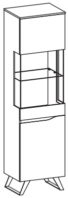
MA-W1/2 witryna L,P W:2000 S:548 G:420
